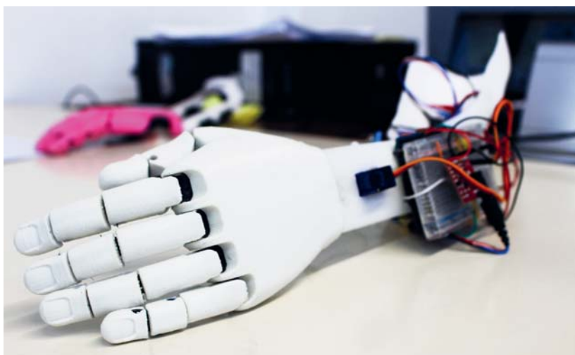
Modelo de prótesis de mano mioeléctrica.
